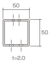
支柱断面図
