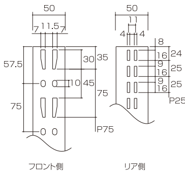
支柱詳細図
